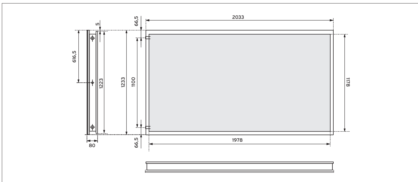
Schéma s rozměry VFK 135/3 D
