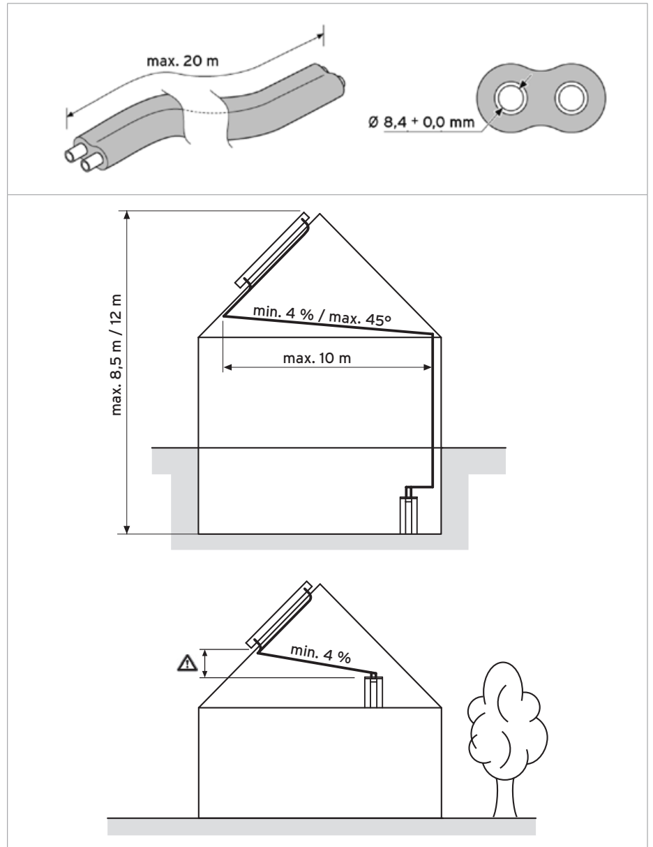
Poznámky k položení potrubí
