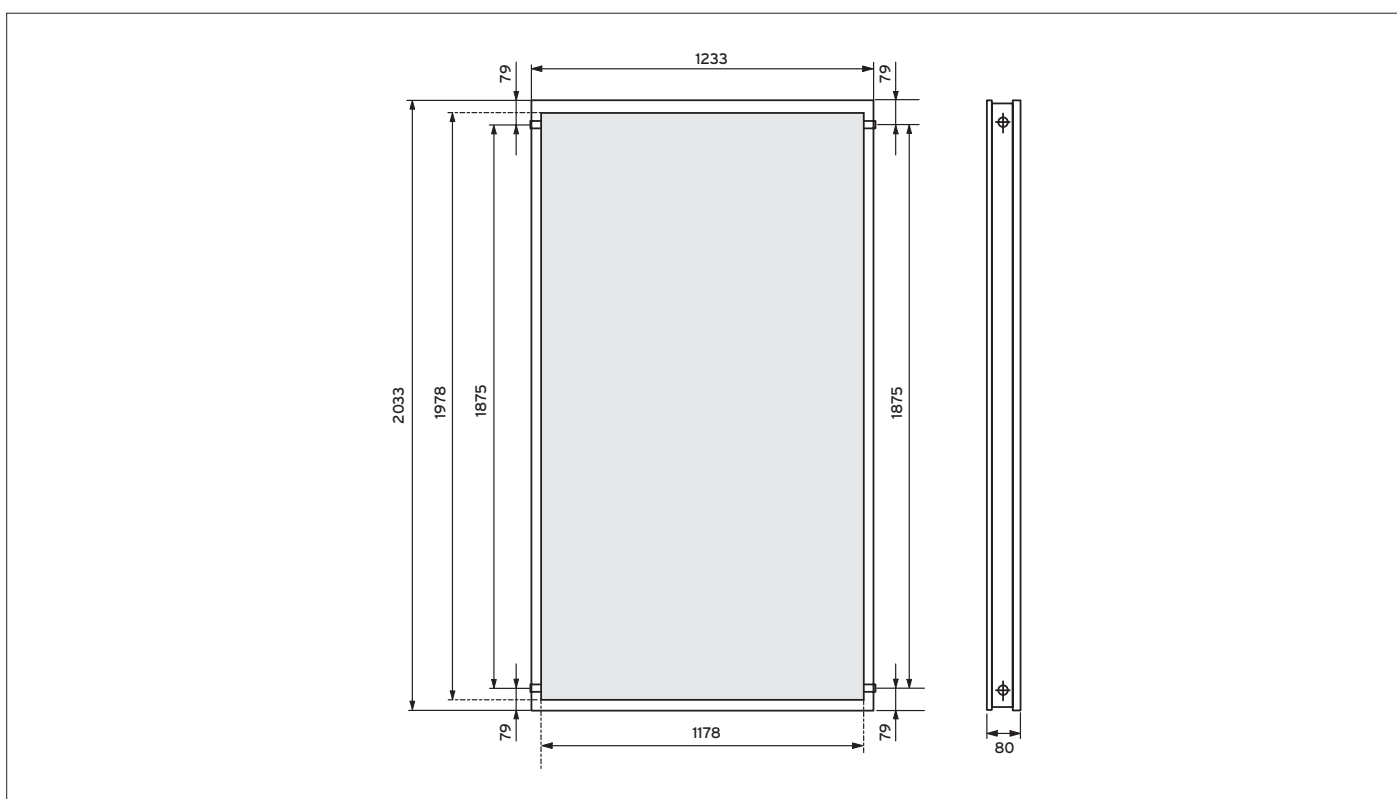
Schéma s rozměry VFK 135/3 VD
