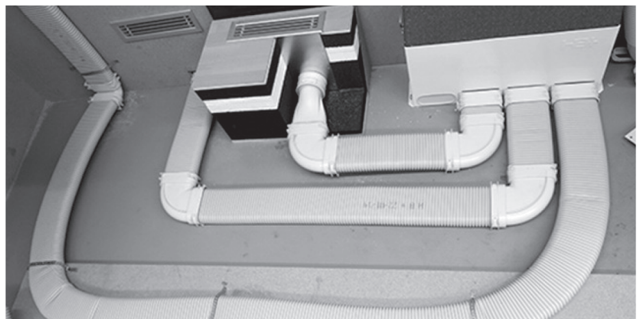
Příklad montáže plochých kanálů
