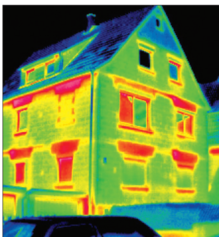
Termografie budovy
