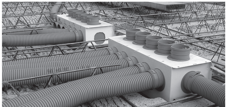
Příklad montáže kruhových kanálů
