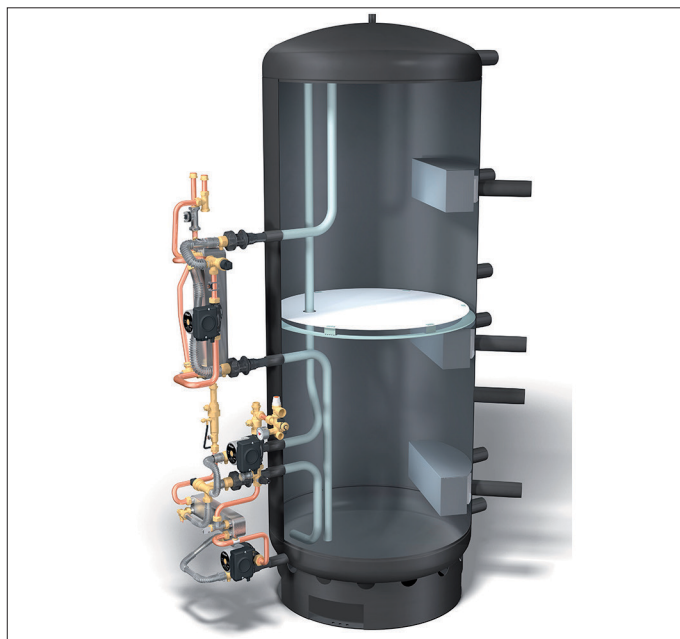
Průřez zásobníkem allSTOR exclusive
