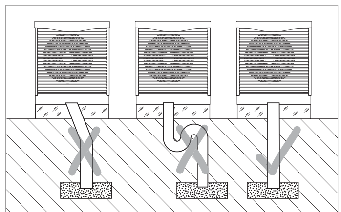
Položení potrubí na odvod kondenzátu
