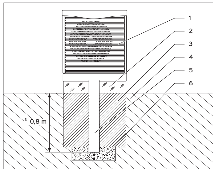
Průřez základů
