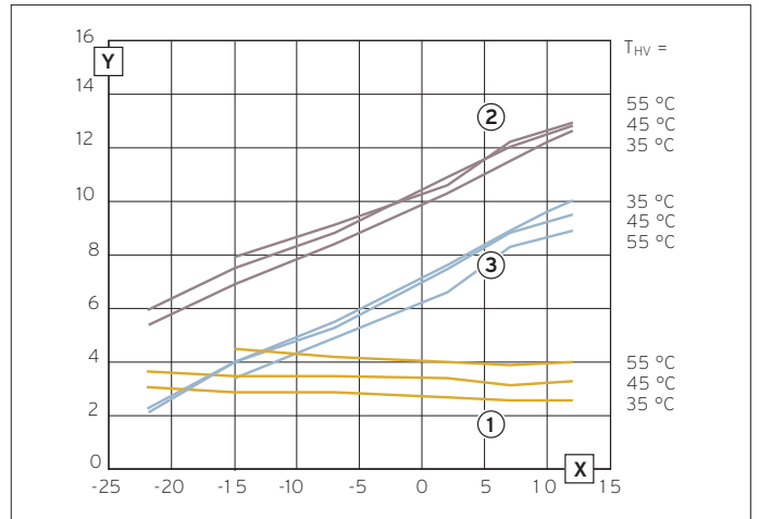
Graf výkonu VWF 118/4
