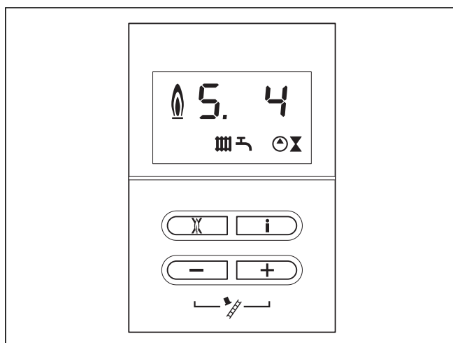
Obr. 9.1 Zobrazení stavových kódů na displeji
