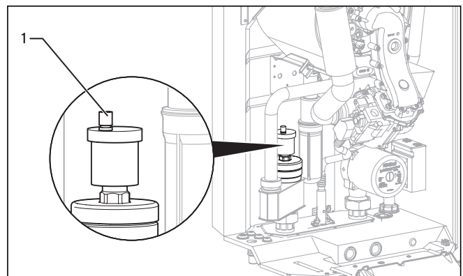
Obr. 6.2 Rychloodvzdušňovač
