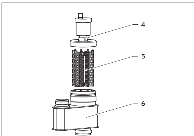
Obr. 8.9 Čištění filtru
