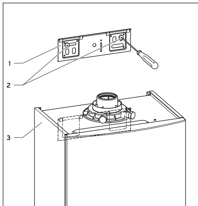
Obr. 4.4 Zavěšení přístroje
