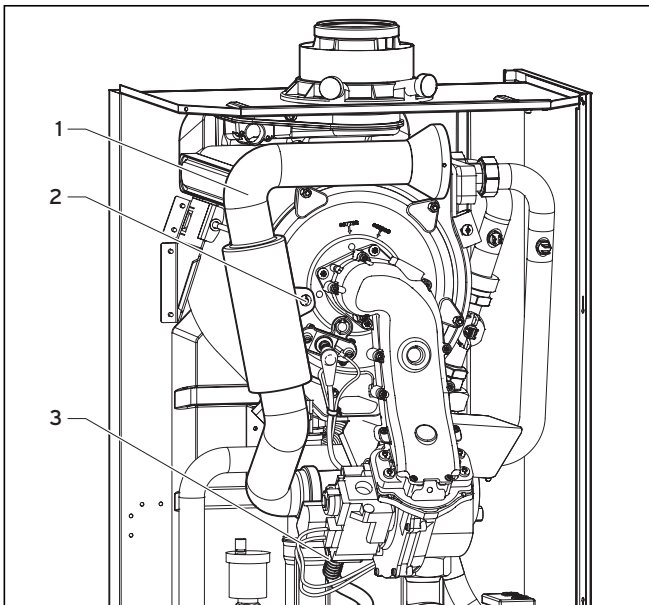
Obr. 8.1 Demontáž potrubí pro sání vzduchu
