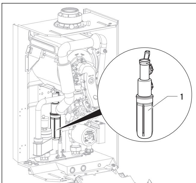
Obr. 8.6 Čištění sifonu pro odtok kondenzátu
