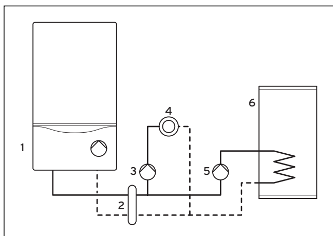
Obr. 5.5 Prioritní obvod zásobníku a topný okruh přes hydraulickou odbočku
