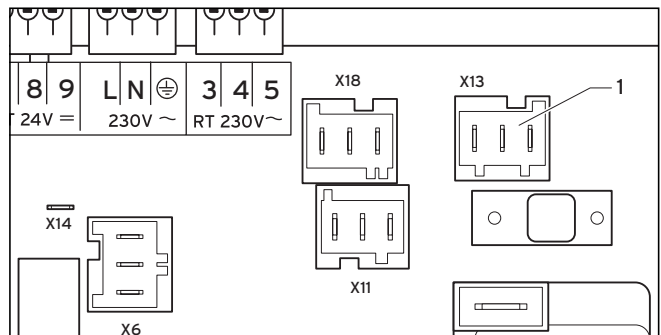
Obr. 5.2 Elektrické zapojení topného čerpadla za hydraulickou odbočkou
