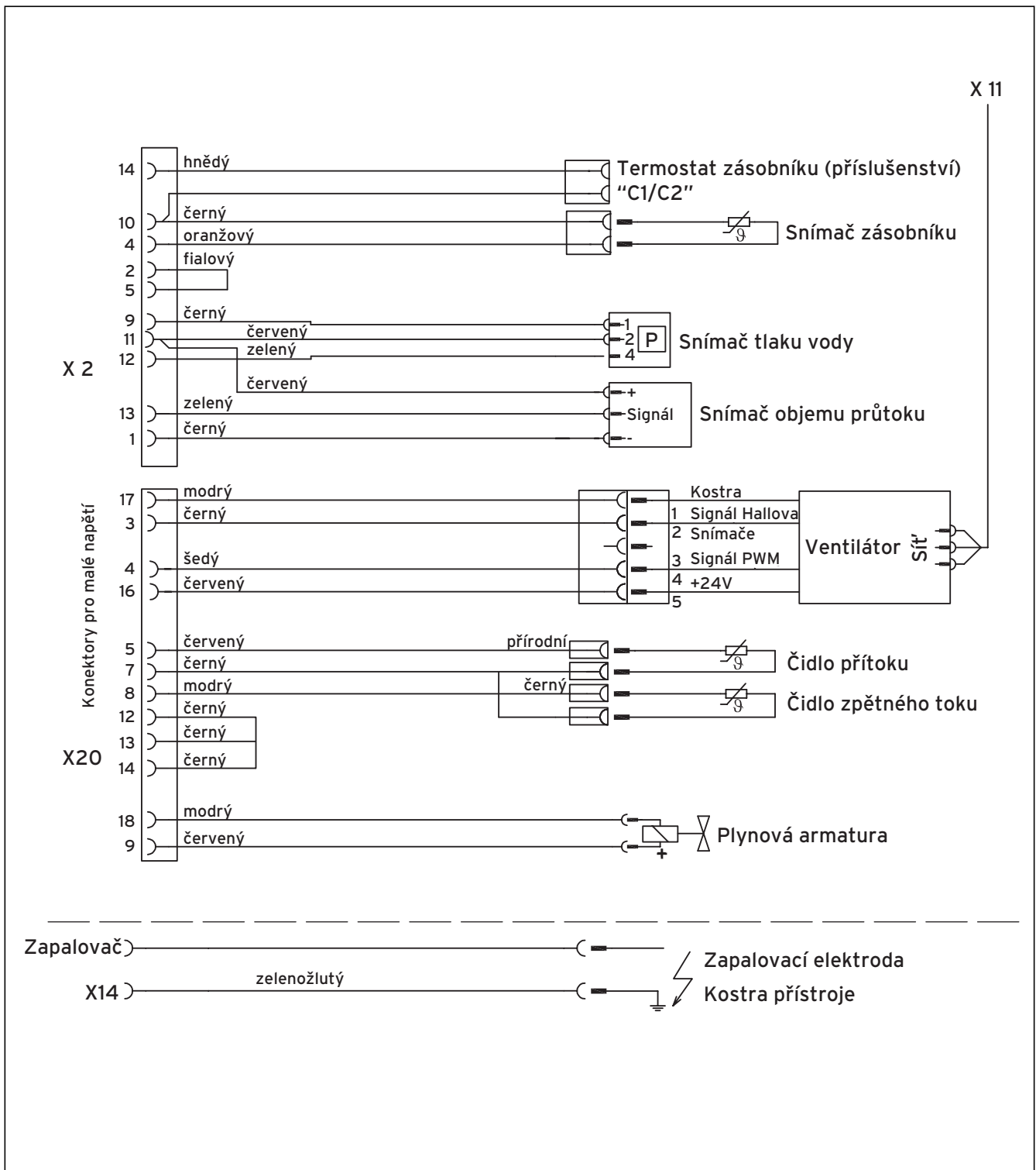
Obr. 5.14 Schéma zapojení zařízení ecoTEC plus (pokr. na další straně)
