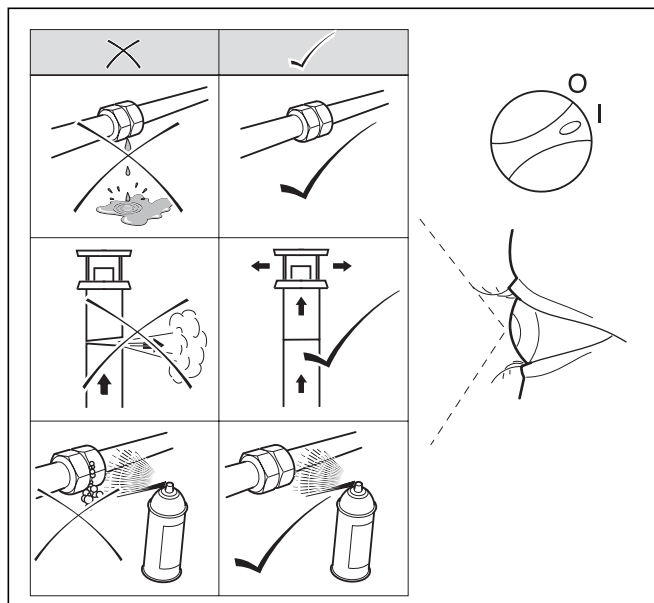
Obr. 8.10 Kontrola těsnosti
