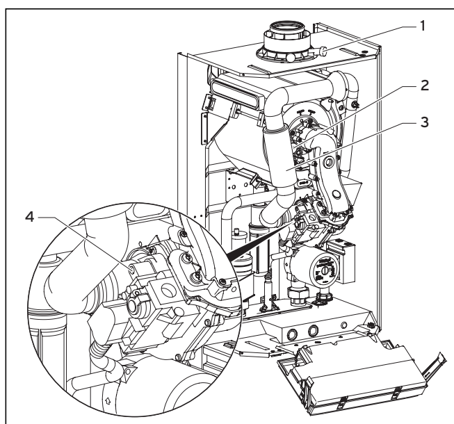
Obr. 6.5 Měření obsahu CO 2 , nastavení poměru vzduchu (nastavení plynu)
