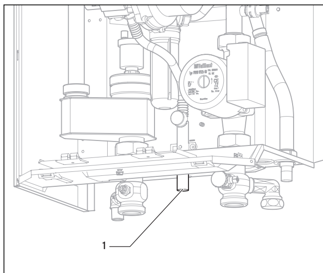
Obr. 5.7 Montáž plynové přípojky
