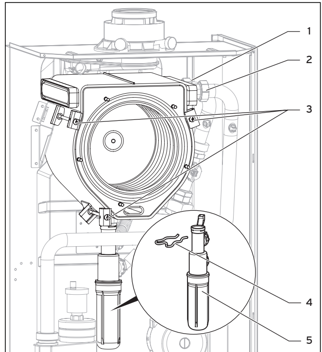
Obr. 10.4 Výměna integrálního kondenzačního výměníku tepla
