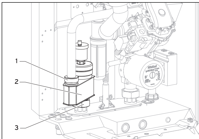
Obr. 8.8 Čištění systému pro odlučování vzduchu
