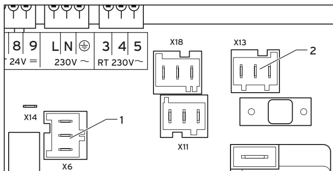
Obr. 5.6 Elektrické zapojení čerpadla pro ohřev zásobníku a externí topné čerpadlo
