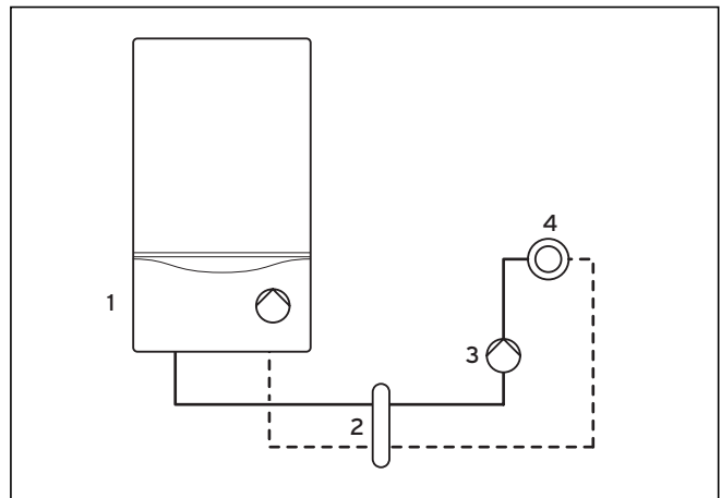
Obr. 5.1 Napojení topného okruhu s hydraulickou odbočkou
