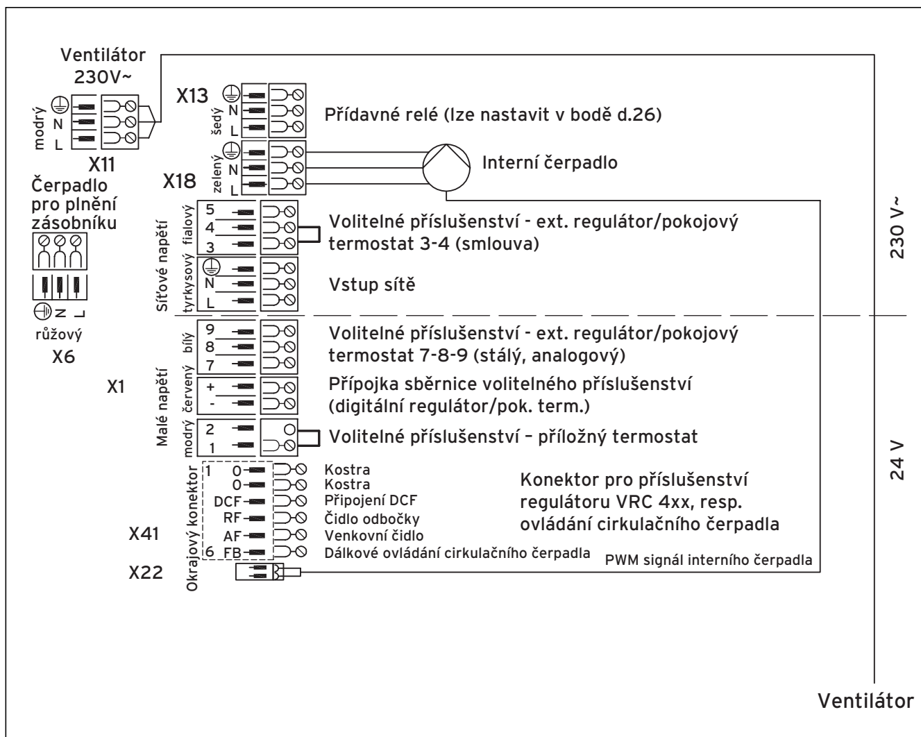
Obr. 5.14 Schéma zapojení zařízení ecoTEC plus (pokrač.)
