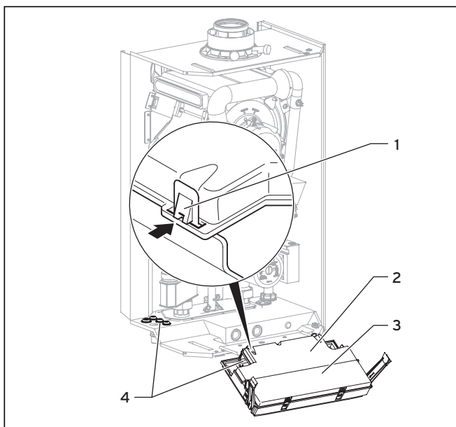
Obr. 5.12 Otevření zadní stěny elektronického boxu
