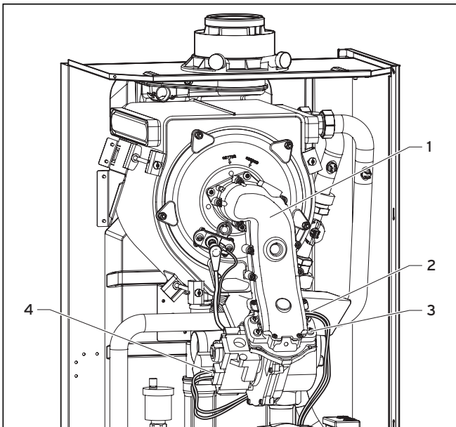
Obr. 10.2 Demontáž ventilátoru s plynovou armaturou
