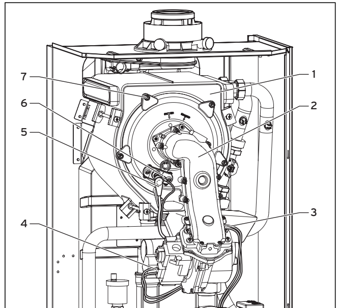
Obr. 8.2 Demontáž termo-kompaktního modulu
