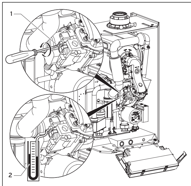
Obr. 6.4 Měření vstupního tlaku (tlak průtoku plynu)
