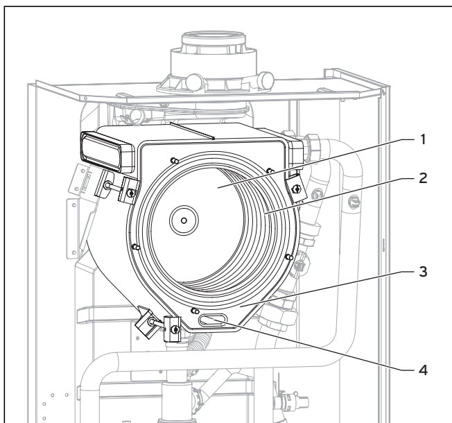
Obr. 8.3 Čištění integrovaného kondenzačního tepelného výměníku
