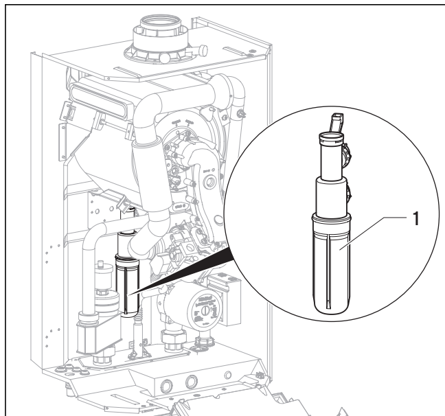
Obr. 6.3 Plnění sifonu pro odtok kondenzátu
