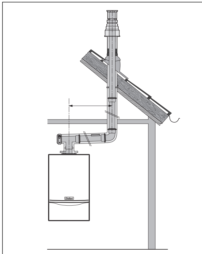
Obr. 5.11 Příklad montáže vertikální střešní průchodky
