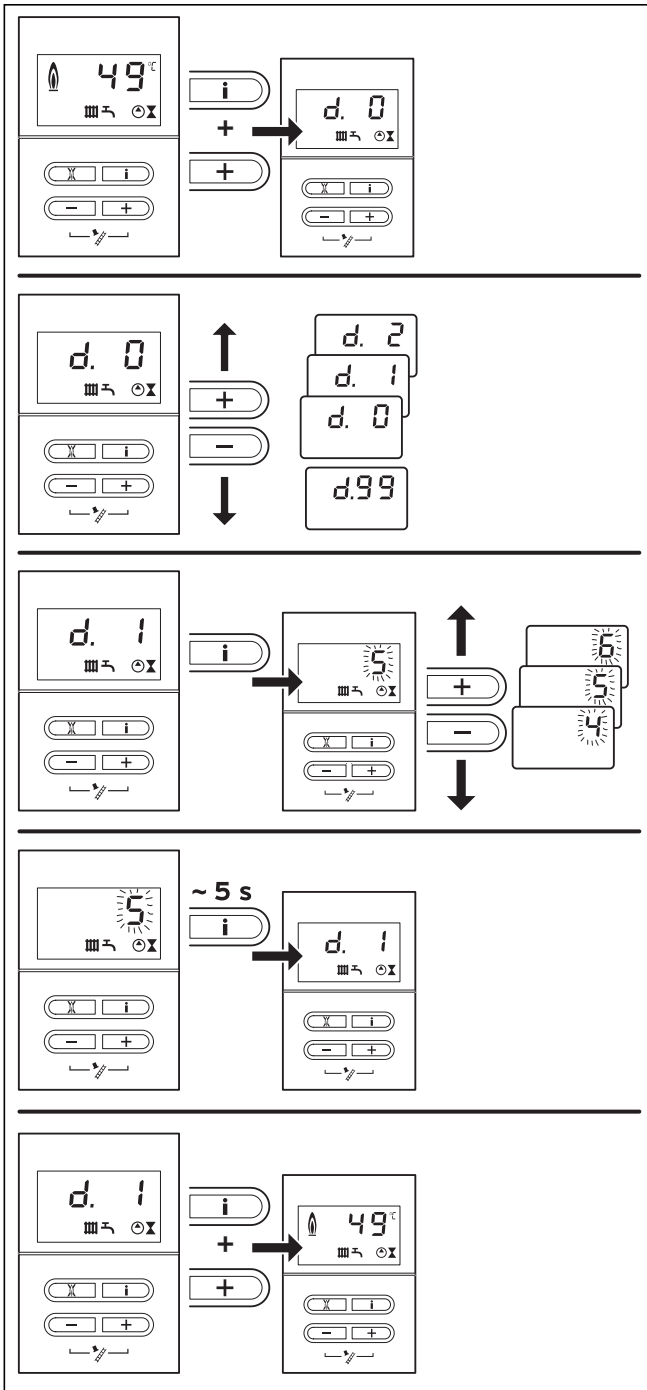
Obr. 7.1 Nastavení parametrů
