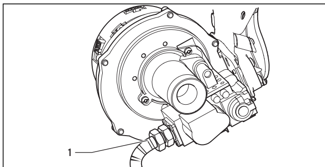
Obr. 8.5 Kontrola plynotěsnosti
