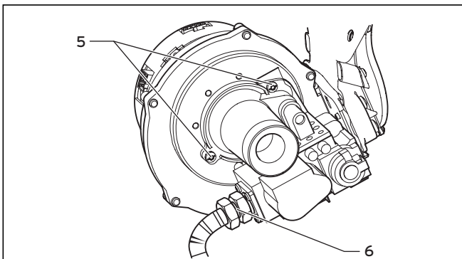
Obr. 10.3 Šroubové spoje plynové armatury/ventilátoru
