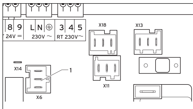
Obr. 5.4 Elektrické zapojení čerpadla pro ohřev zásobníku
