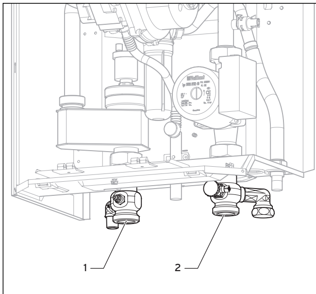
Obr. 5.8 Připojka topení
