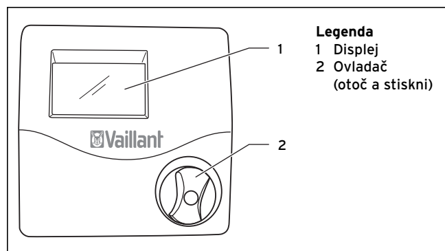
Obr. 1.1 Přehled zařízení
