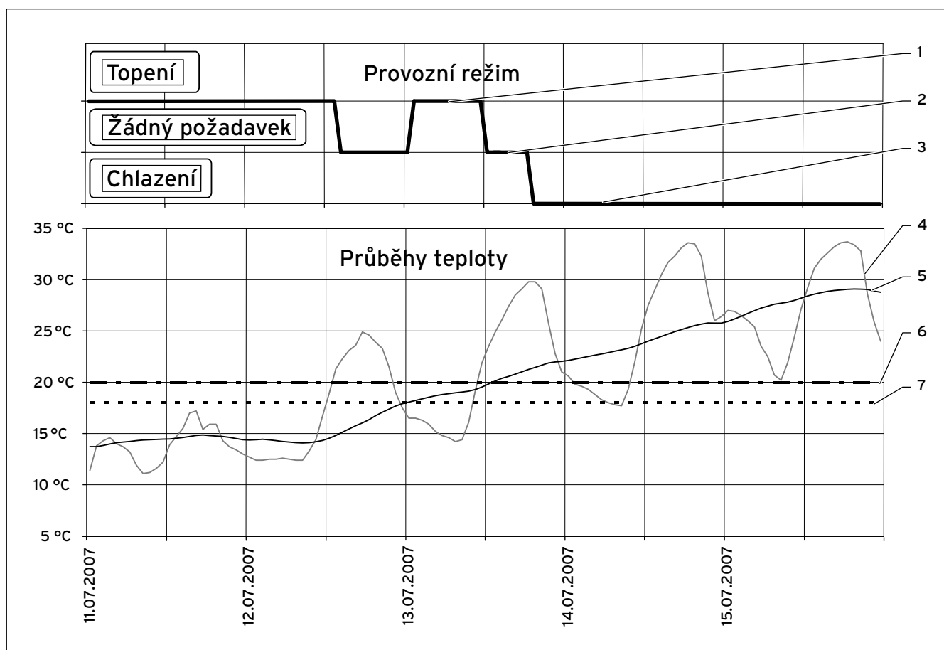
3.5 Příklad přepínání mezi topením a chlazením podle venkovní teploty
