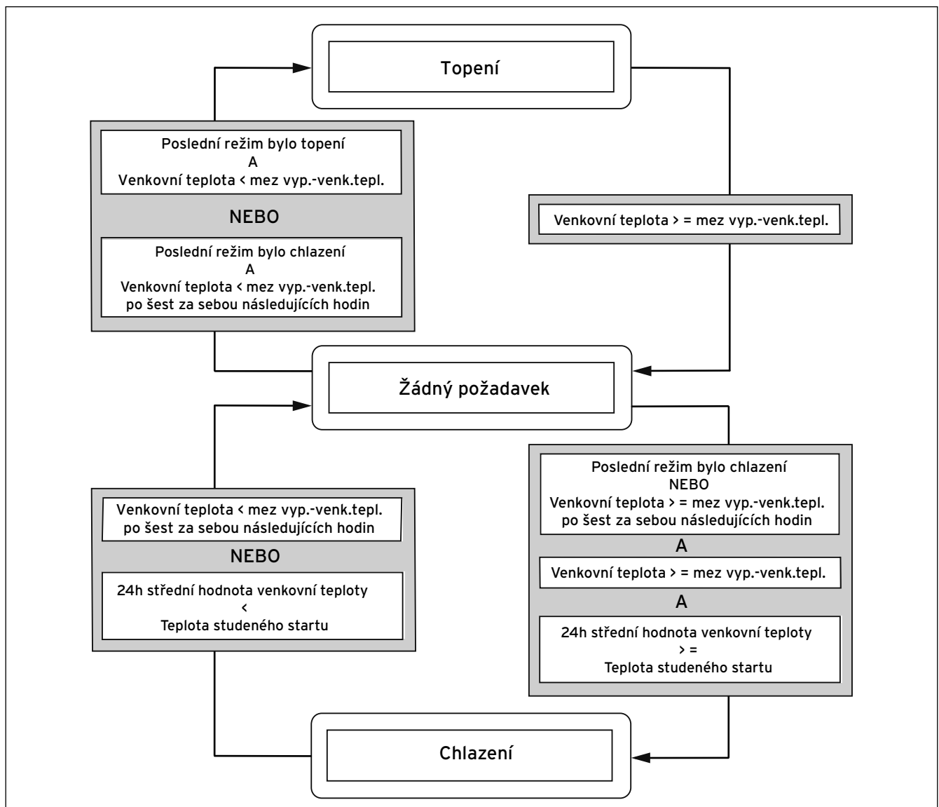
3.4 Přechodové schéma
